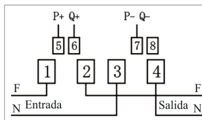
Fig. 3: Terminales del medidor
