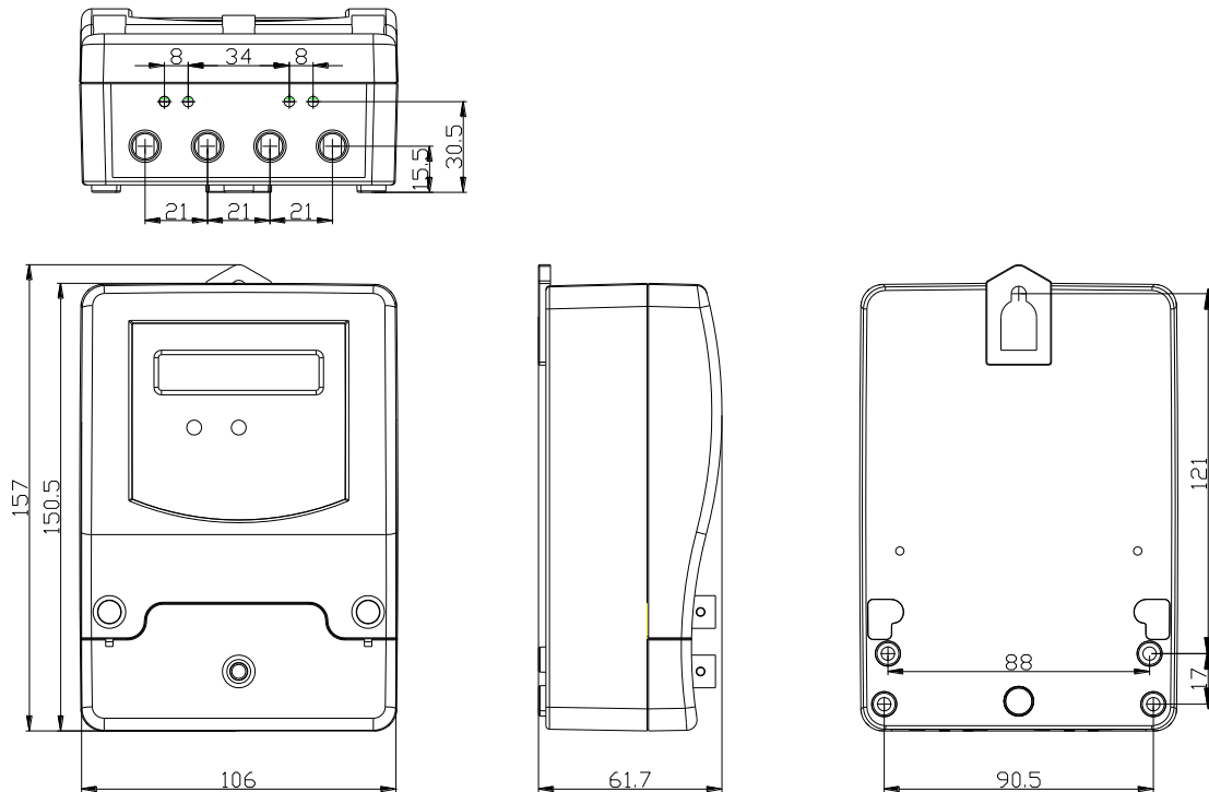
Fig. 2 Dimensiones del medidor.
